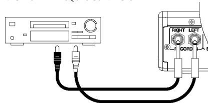
SORTIE LIGNE
